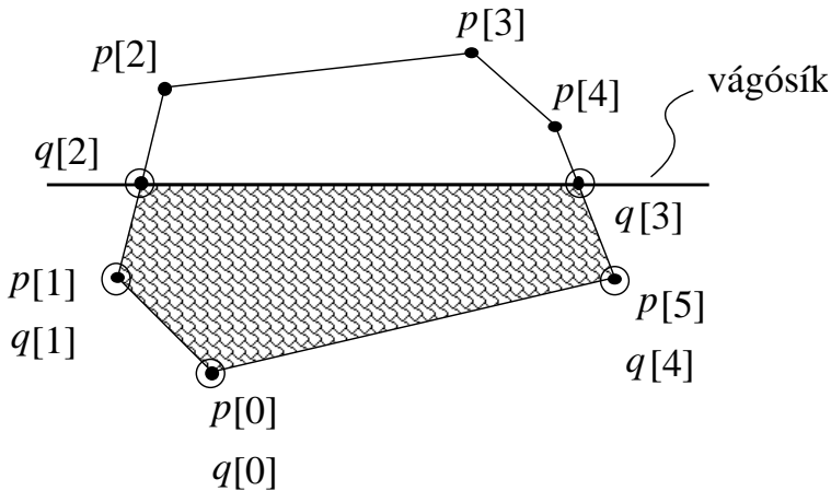
40.26. ábra. A \vec{p}[0], \dots, \vec{p}[5] sokszög vágása, amelynek eredménye a \vec{q}[0], \dots, \vec{q}[4] sokszög. Az eredmény sokszög csúcsai az eredeti sokszög belső csúcsai és az élnek a vágósíkkal képzett metszéspontjai.
