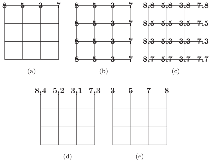
3.12. ábra. Ritka leszámlláló rendezés négyzeten
